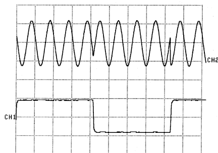
CH1 → Modulationssignal CH2 → Moduliertes Signal (Frequenzhub: 1 rad)
